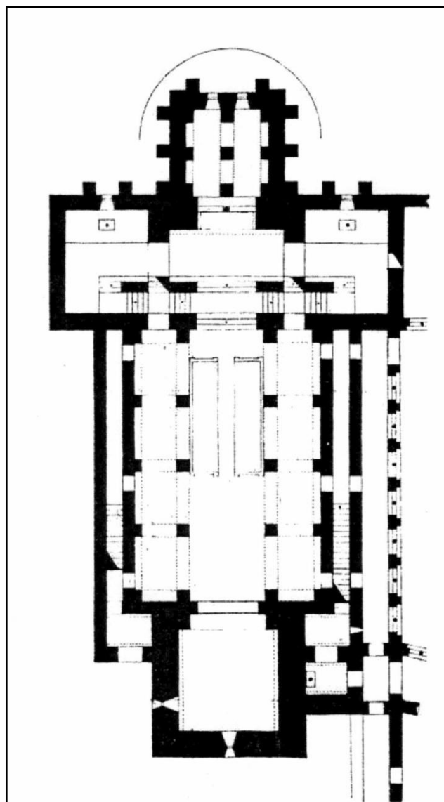
Fig. 1a - Plan idéal de "Gellone I" (1 er niveau : parties existantes et parties reconstituées), 802-805. La salle basse du Westwerk (probable Panthéon) se trouve au fond de la nef centrale. La Cellule de Guilhem est plaquée au S.
