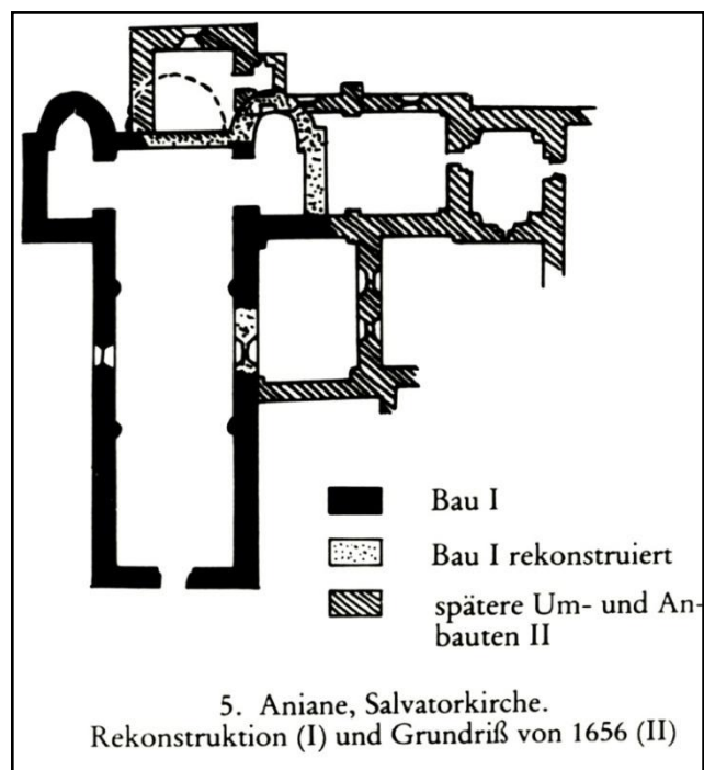
Fig. 6 - Aniane, église carolingienne (d'après B.Uhde-Stahl in Zeitschrift für Kunstgeschichte , t. XLIII, 1980, fig. 5, p. 5).
