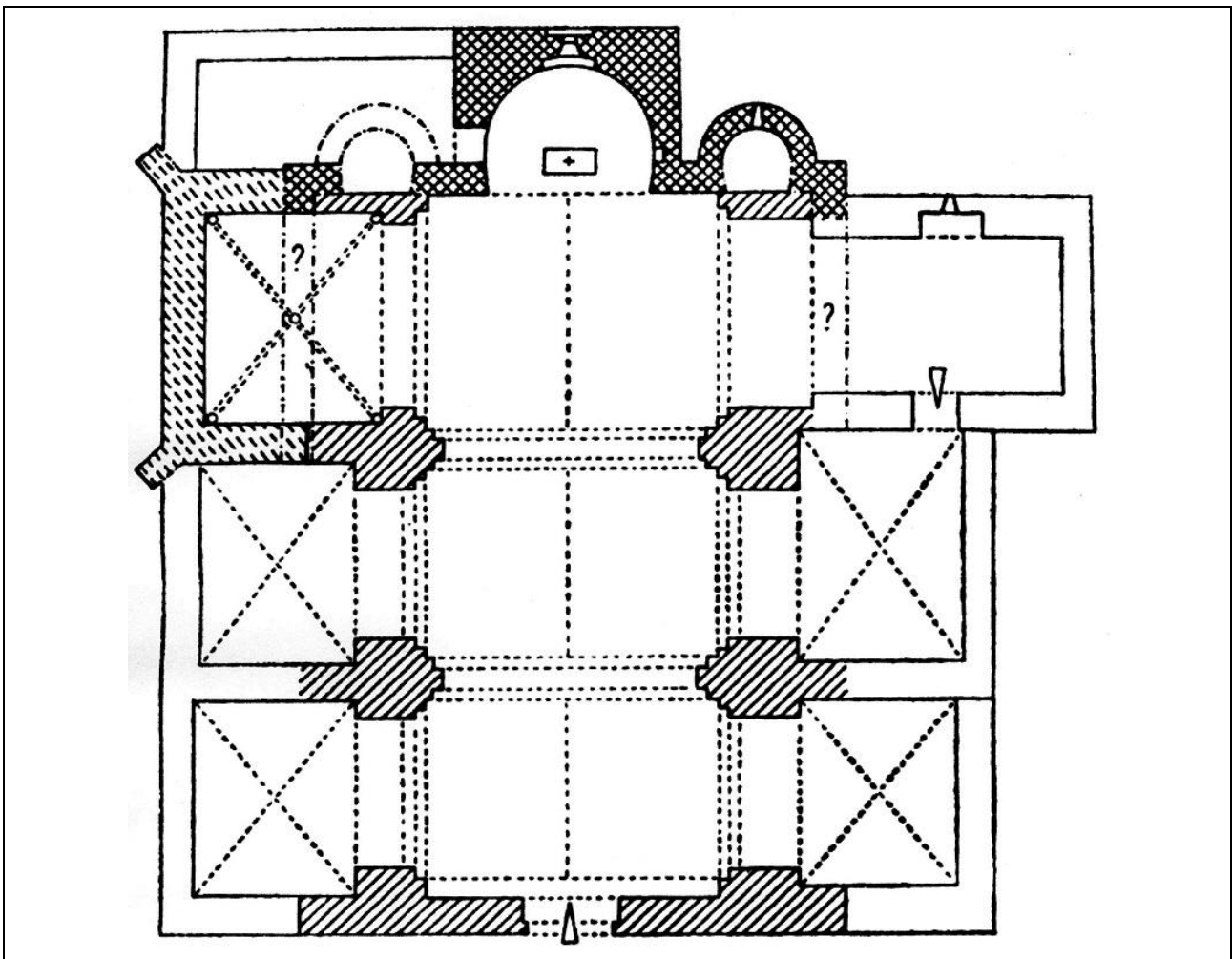
Fig. 8 - Vaugines, plan après 1004 (d'après Dom Noël Deney, in G. Barrauol, Provence romane 2. La Haute-Provence , p. 90).
