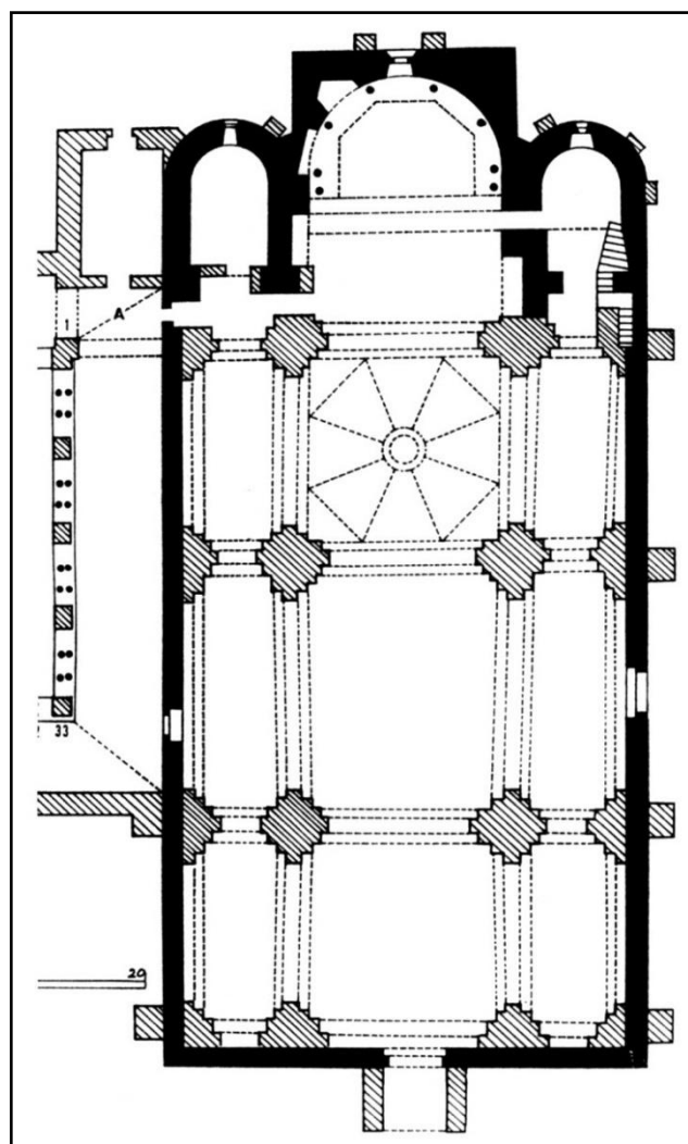
Fig. 5 - Vaison-la-Romaine, cathédrale (d'après Dom Noël Deney, in J.-M. Rouquette, Provence romane. La Provence rhodanienne, p. 144).
