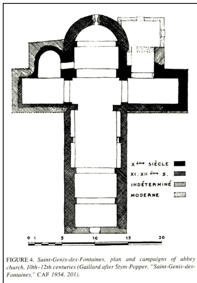
Fig. 7 - Saint-Genis-des-Fontaines (d'après S. Stym-Popper, "Saint-Genis-des-Fontaines". Congrès archéologique de France , 1954, p. 201).
